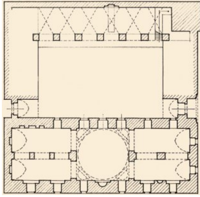
Cammi Planı
